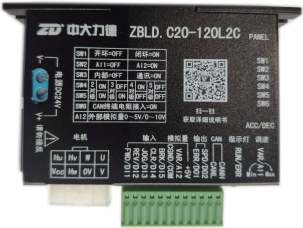
驱动器本体
